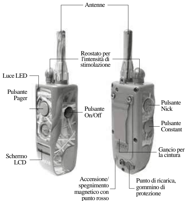
Trasmettitore
