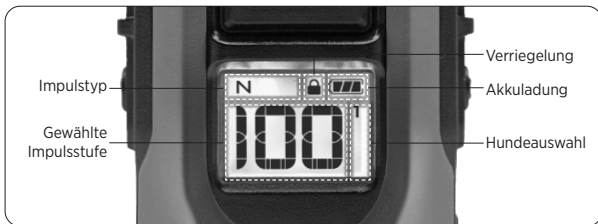
ARC-X LCD-Bildschirm des Senders
