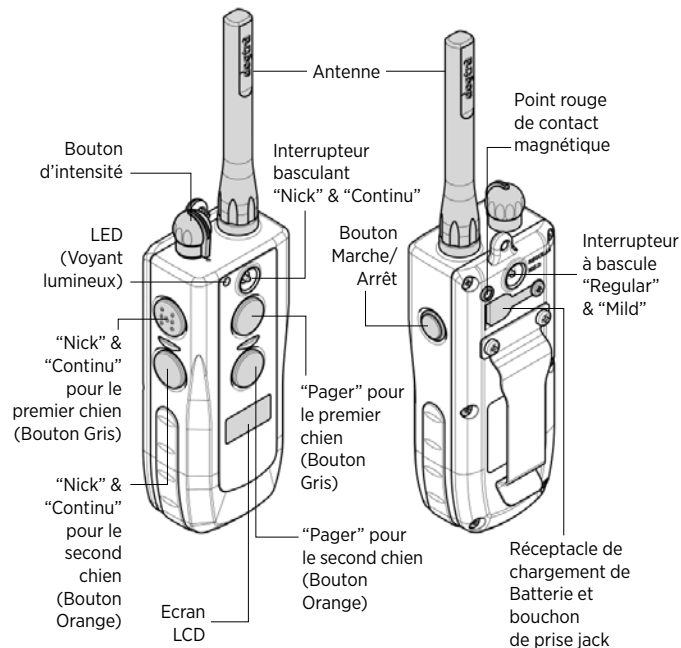
3500NCP Emetteur
