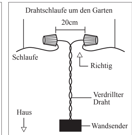
Richtige Drahtverbindung
